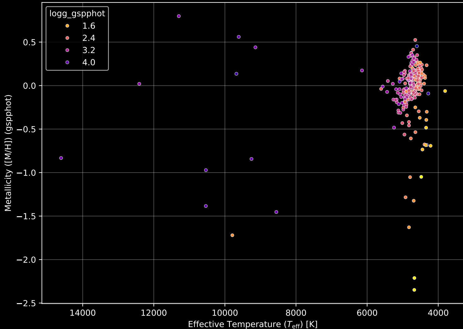
APOGEE DR17 Field: [049-06] Stellar Population Parameters (n= 281)
